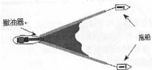
图 5-3 三船开口 U 形布放围油栏
