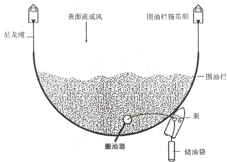
图 5-9 二船拖曳围油栏成"U"形
