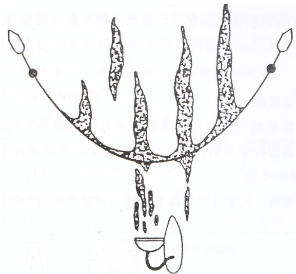
图 5-10 二船拖曳围油栏成"U"形，逃逸的油用单船收油系统回收
